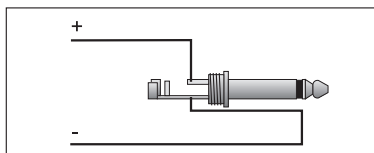
Fig. 2.3: Collegamento ad un'uscita amplificatore
