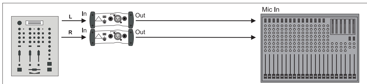
Fig. 2.2: Mixer DJ → 2x Box DI → banco di mixaggio
