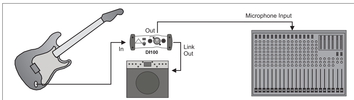
Fig. 2.1: Chitarra → DI-Box → Amplificatore di chitarra / banco di mixaggio
