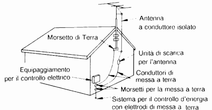
Esempio di messa a terra dell'antenna
