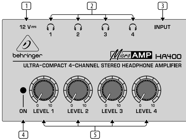
Elementi di comando ed attacchi del HA400
