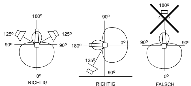
PLAZIERUNG UNERWÜNSCHTER SCHALLQUELLEN
