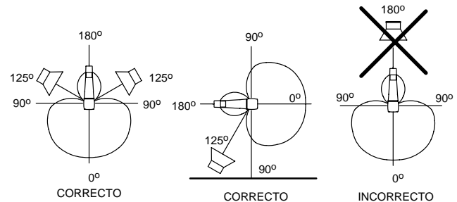
COLOCACION DE FUENTES SONORAS NO DESEADAS
