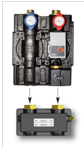
Separatore idraulico 60/80 Adatto al montaggio diretto alle stazioni pompa oppure ai collettori di distribuzione
